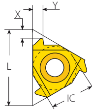
Aussen Standard
