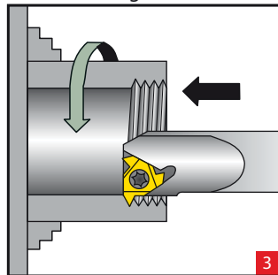
Innen- Rechtsgewinde
