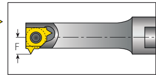
Mini-L-Gewinde
