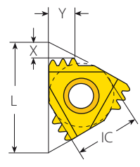
M+ Typ
