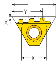
T+ Typ
