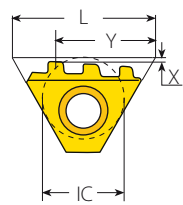
T+ Typ
