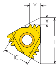
M+ Typ
