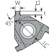
Standard (Vollprofil)
