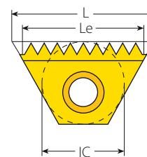
Regelgewinde TM
