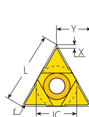
U Typ
