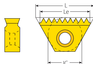
Regelgewinde TM
