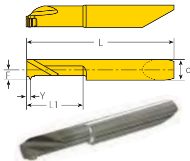
RH - Einseitig
