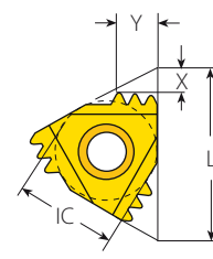
M+ Typ
