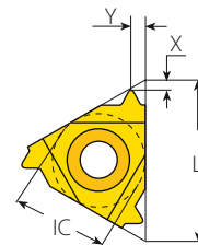
Innen - Norm
