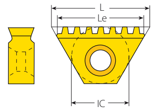
Regelgewinde TM
